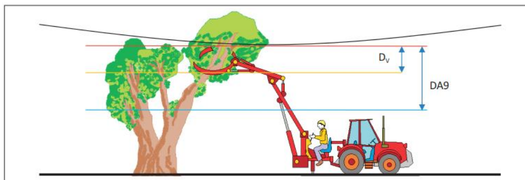
Fig. 14: Attrezzatura di lavoro con lavoratore in situazione di pericolo.
