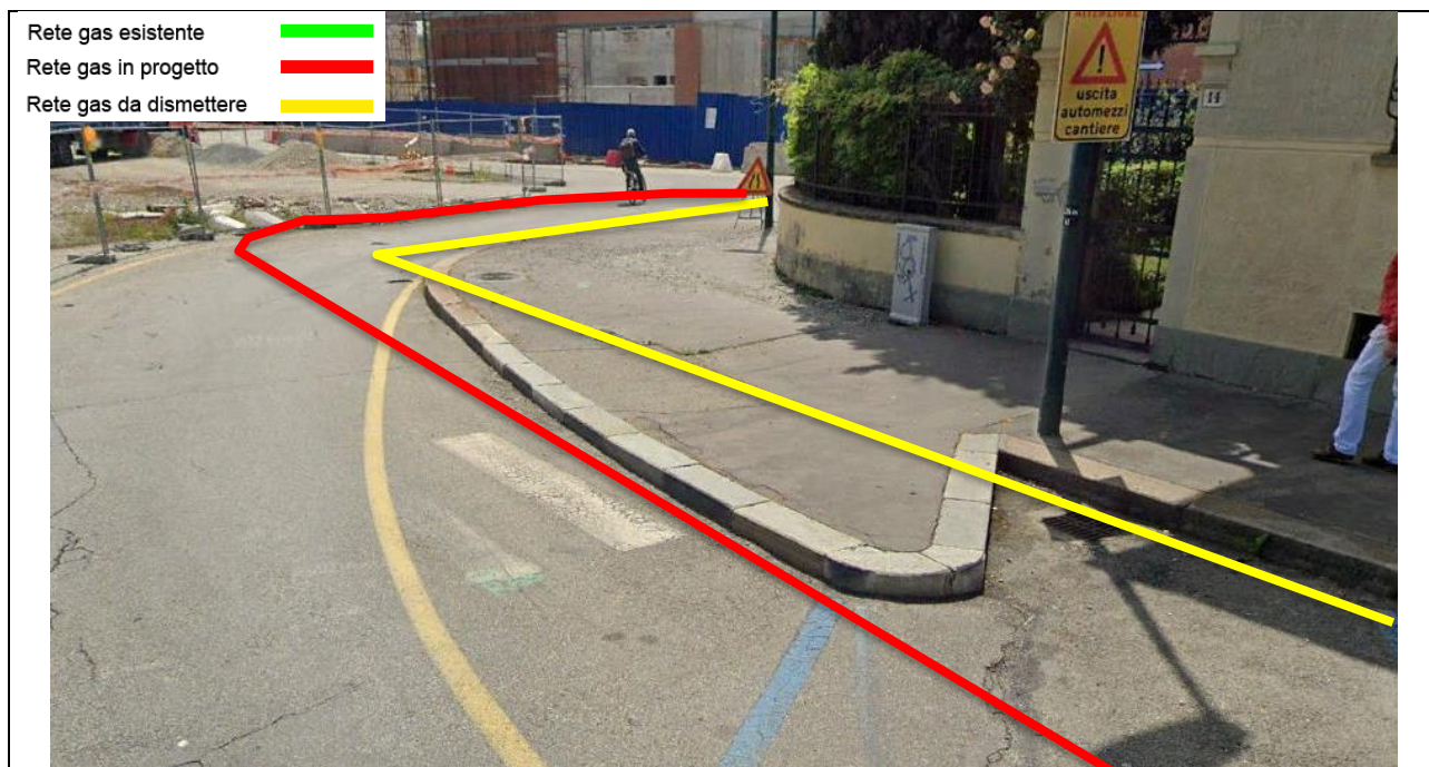
Foto 4 – Proseguimento condotta Via Camogli direzione Via Carlo Forlanini
