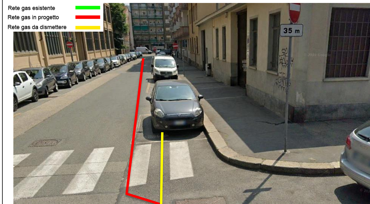
Foto 13 – Stacco condotta Via Busca
