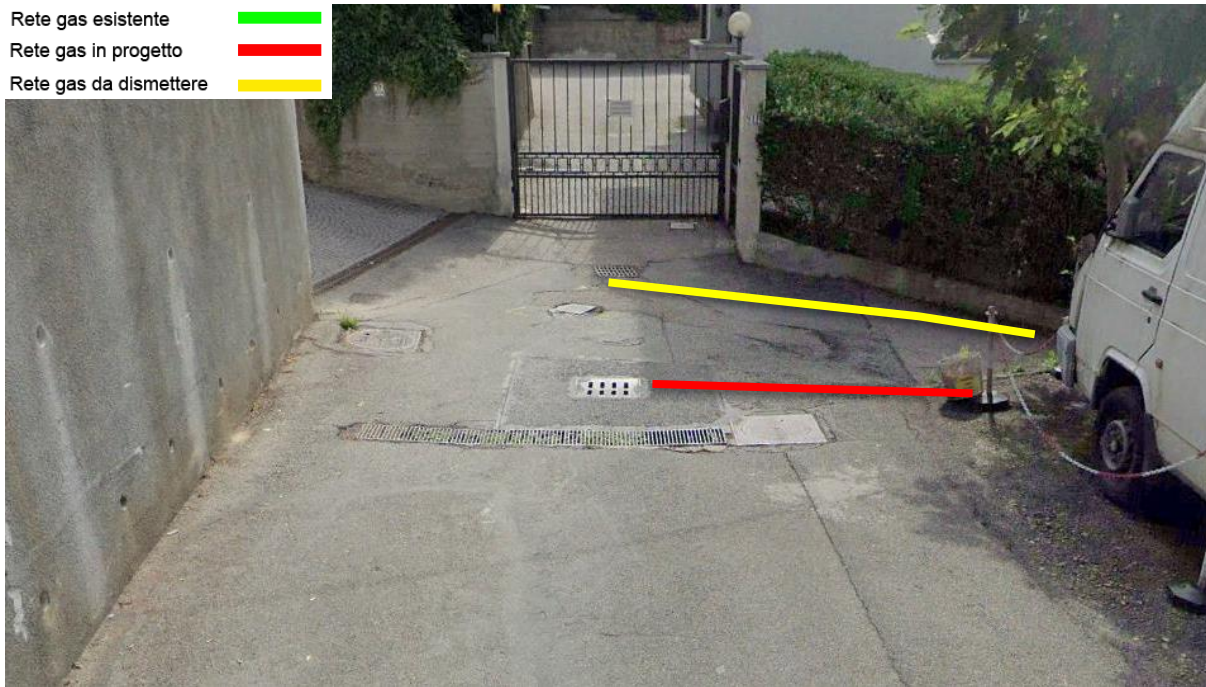
Foto 65 – Stacco condotta Str. Sappone
