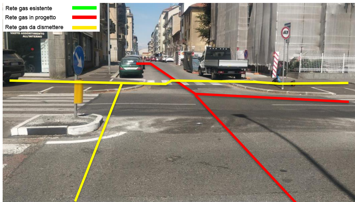
Foto 54 – Percorrenza condotta Via Caramagna derivazione Via Sommariva
