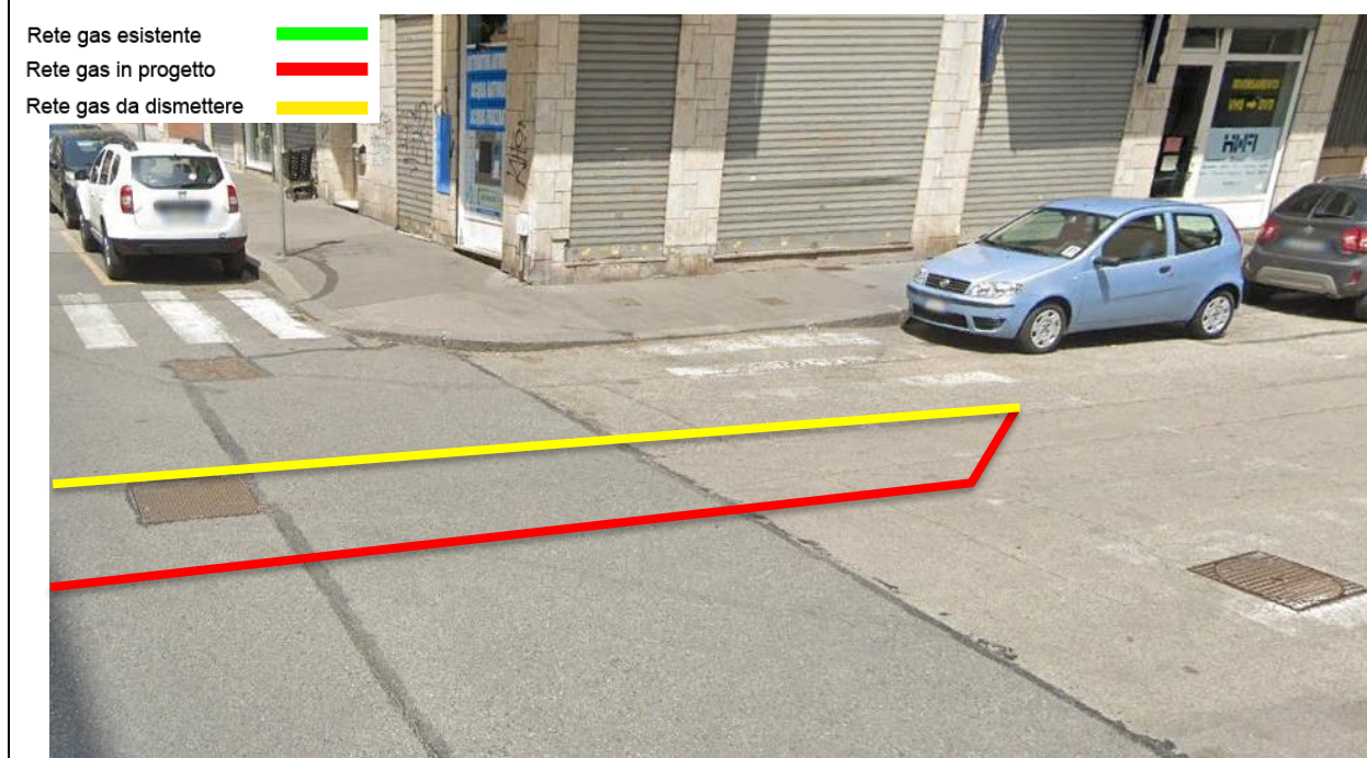
Foto 60 – Percorrenza condotta Via Testona derivazione Via Barbaresco
