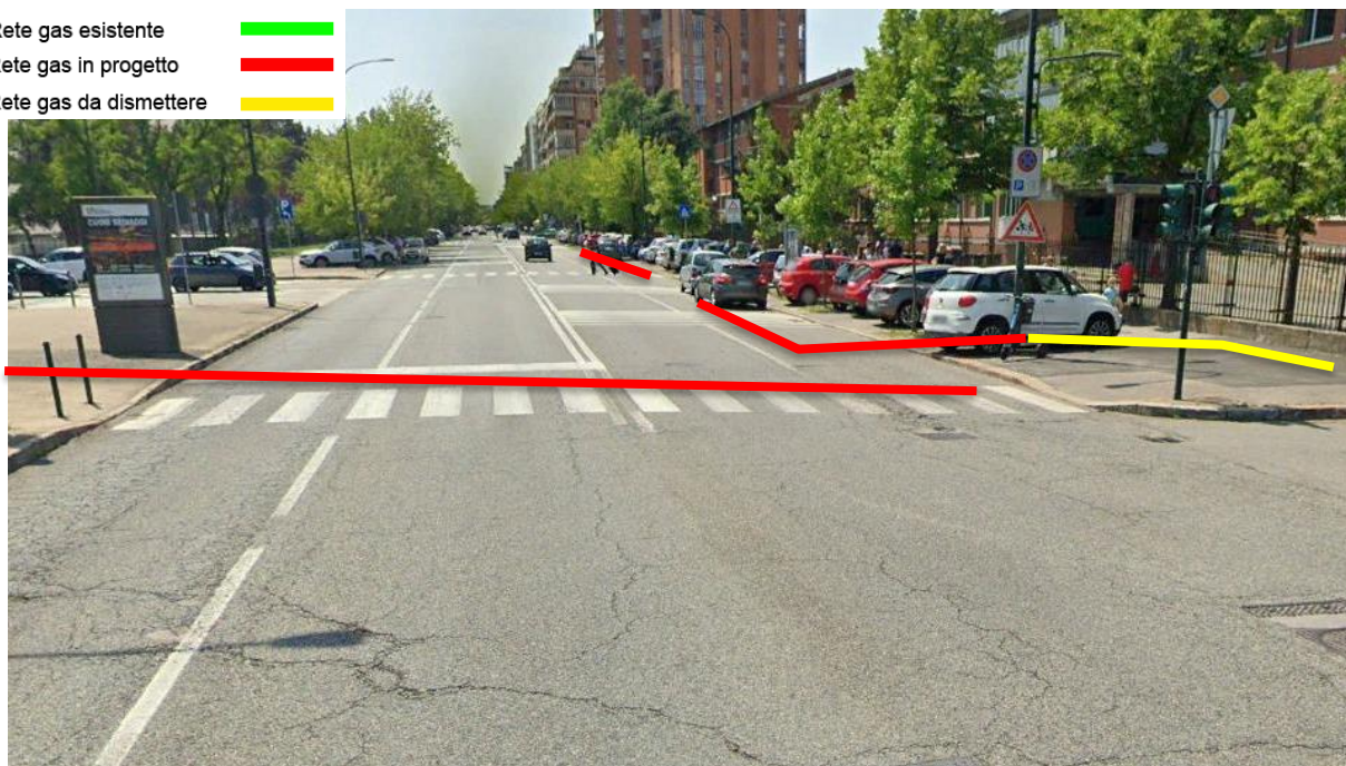
Foto 49 – Stacco condotta Via Ventimiglia
