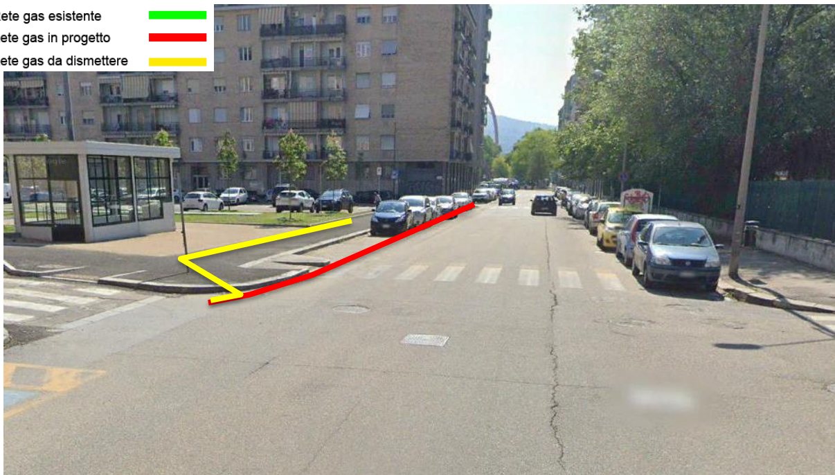
Foto 16 – Stacco condotta Via Asuncion
