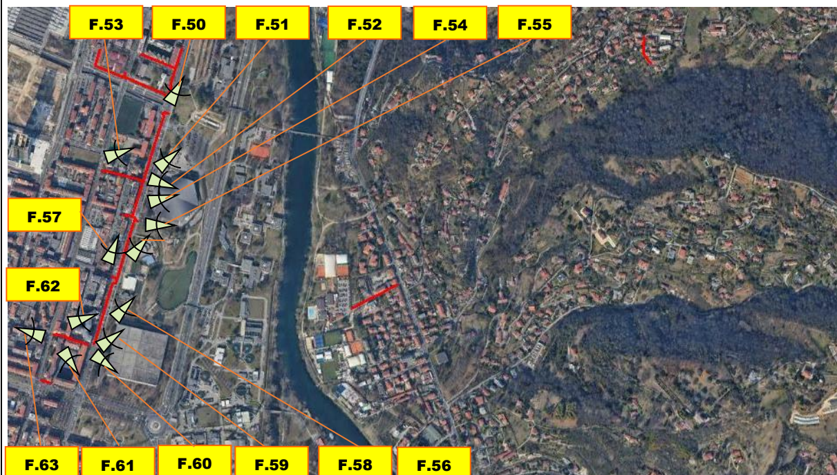
Figura 6: Inquadramento intervento su base ortofoto Area C
